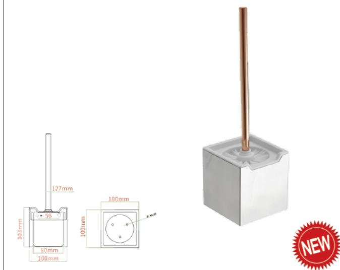
Model: JQS-V007 马桶刷 Toilet brush
