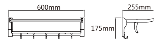
Model: JQS-A845(亮光) B845(砂光) (50cm 60cm) Model: JQS-A850(亮光) B850(砂光) (50cm 60cm) 不带杆
