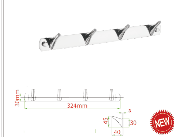
Model: JQS-M010-4 衣钩 Hook
