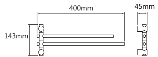
Model: JQS-G2 双杆活动巾杆
