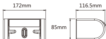
Model: JQS-001 纸架
