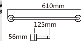
Model: JQS-2513 单毛巾杆 18" 24" 30"
