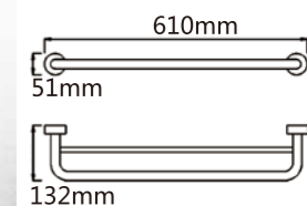
Model: JQS-2513 单毛巾杆 18" 24" 30"
