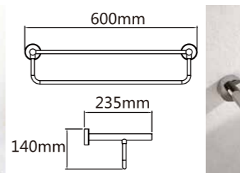
Model: JQS-2508 单毛巾杆 18" 24" 30"
