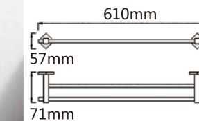
Model: JQS-2313 单毛巾杆 18" 24" 30"
