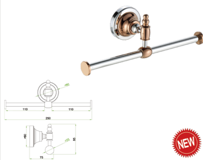
Model: JQS-N005 双纸巾架 Double paper holders
