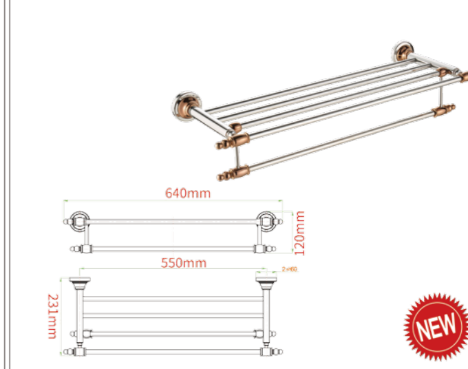
Model: JQS-N008 毛巾架 Towel shelf
