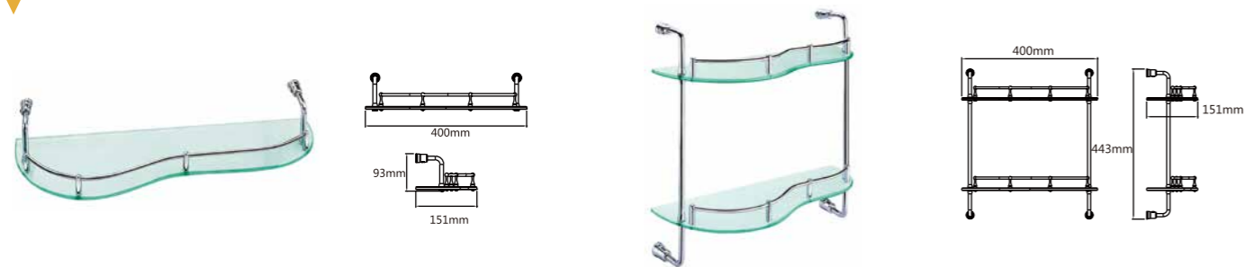
Model: JQS-B1 单层砂玻璃架 (40cm 50cm 60cm)
